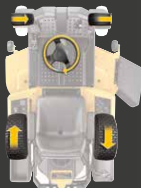
EFFEKTIV 4-HJULSSTYRNING På Z1 / Z5 / Z7 / Z9
